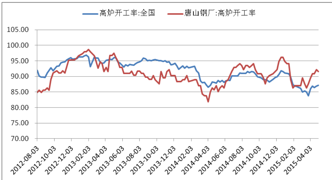
图 8：高炉开工率
